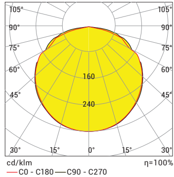
WH154 Ex CW 120D 128W 220V AC
